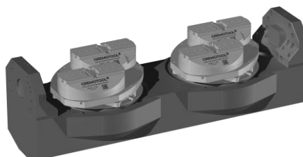
Spannmittel: 4x HMC-120 Vorrichtung: NPS versetzt
